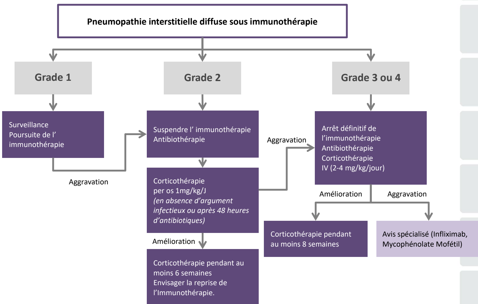
Figure 10 – Proposition d’algorithme décisionnel en cas d’événement indésirable d’ordre respiratoire survenant sous immunothérapie (d’après (124)).
